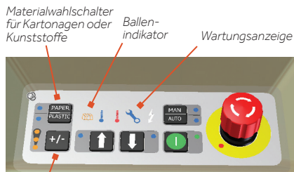
Einstellbare Ballengröße
