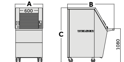
Welger RV642
